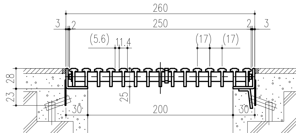
断面図
