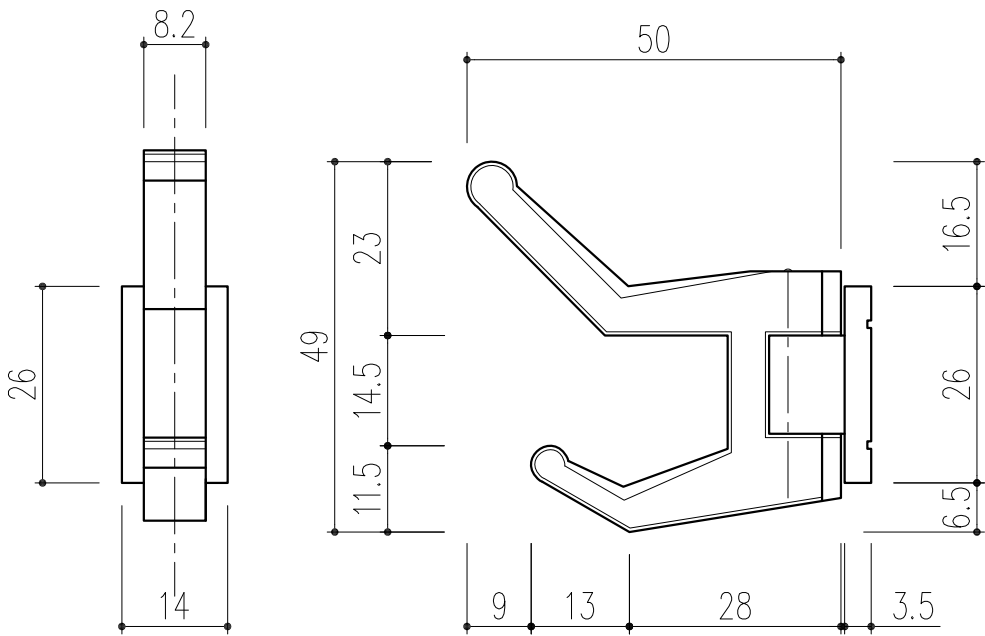
マイティーレイル プラスチックフック
