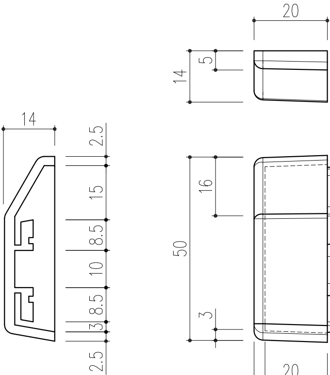
マイティーレイル サイドキャップ
