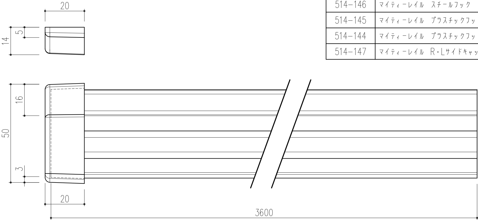
マイティーレイル
