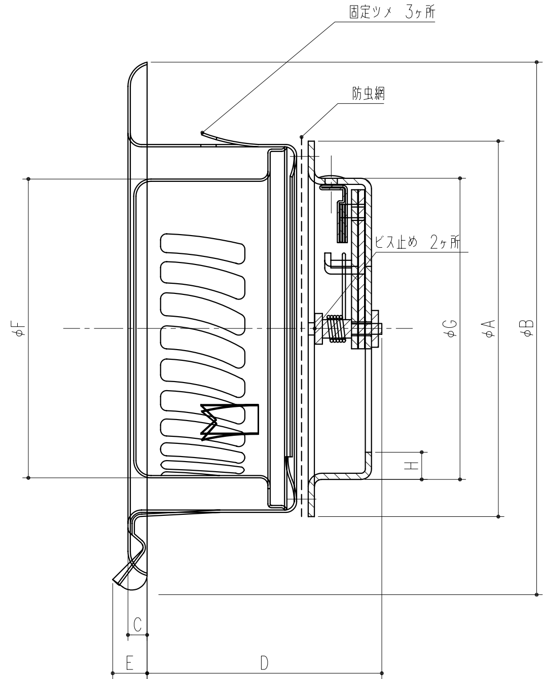
縦断面図
