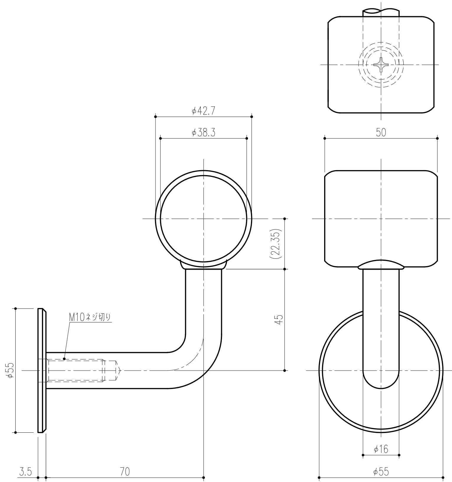
■付属部品 カットアンカー C-1060 : 1本
