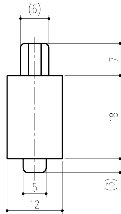
原寸図
