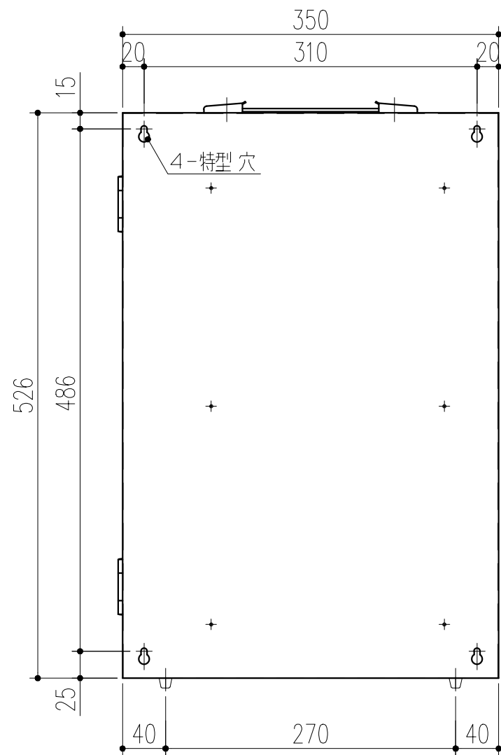
背面図 S=1/5
