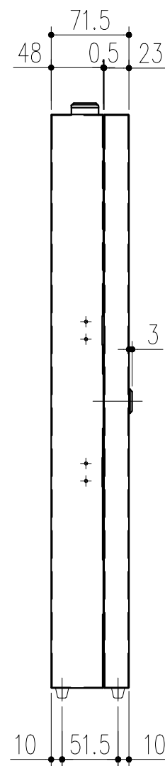
側面図 S=1/5
