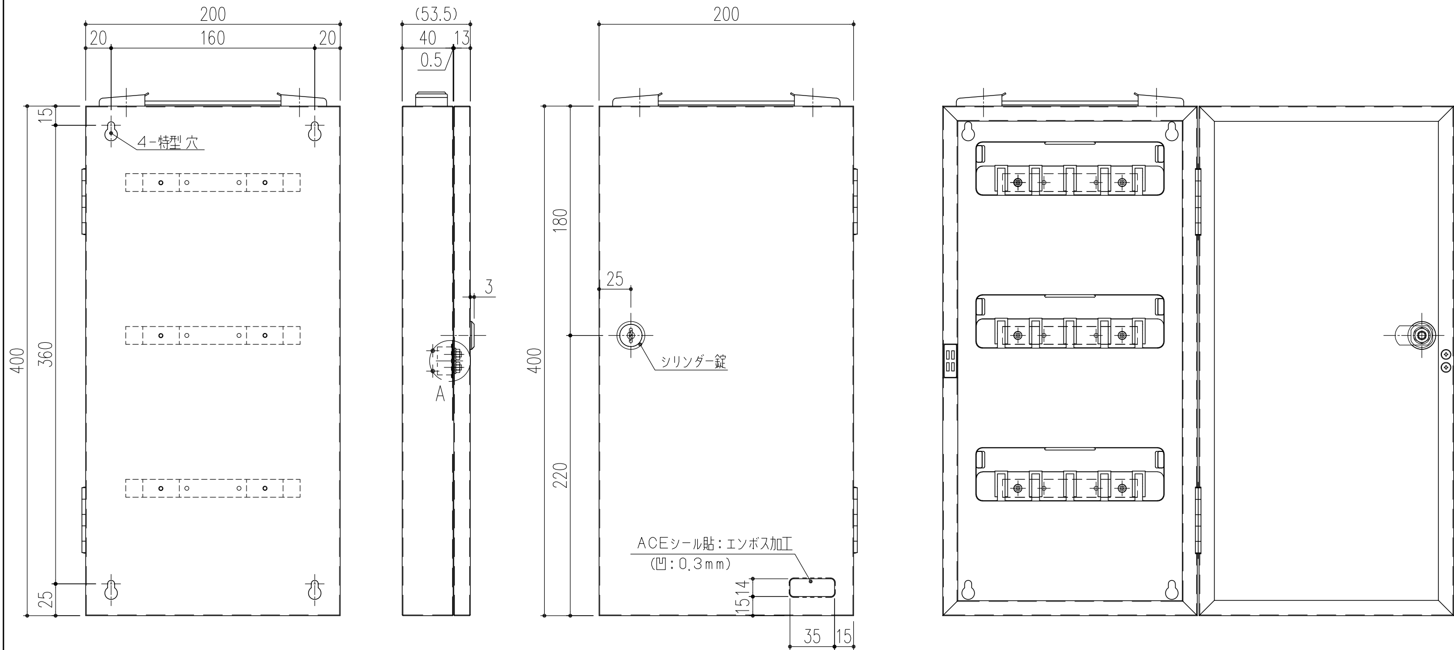
背面図 S=1/3
