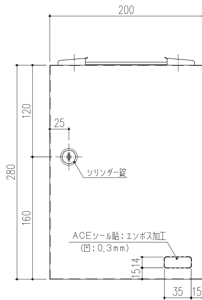
正面図 S=1/3
