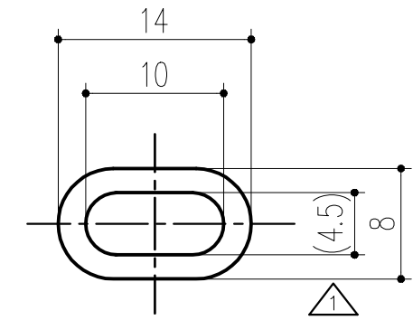
ルースホール詳細 S=2/1
